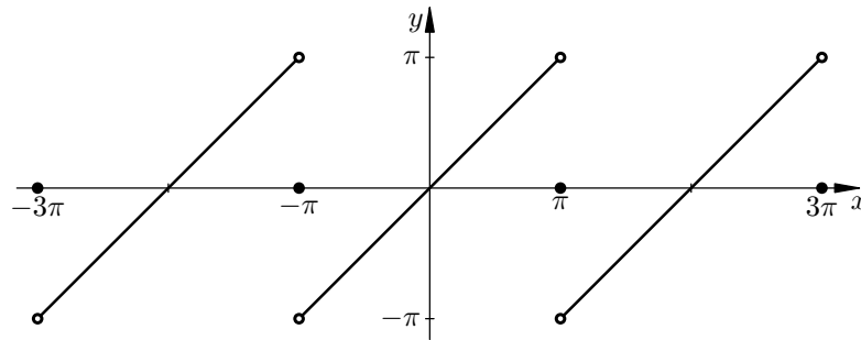
Obr. 4.1: Součtová funkce
